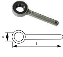
GER/GSK-Spanner
